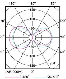
LEDTrueForce E27 360
