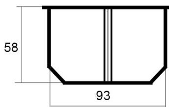
Målskisse
