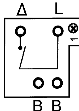
Koblingsskjema
