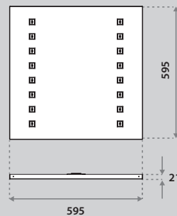
Aviora FL 595x595 (IP20)
