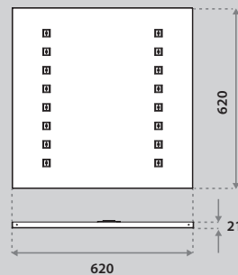
Aviora FL 620x620 (IP20)
