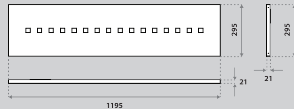
Aviora FL 1195x295 (IP20)
